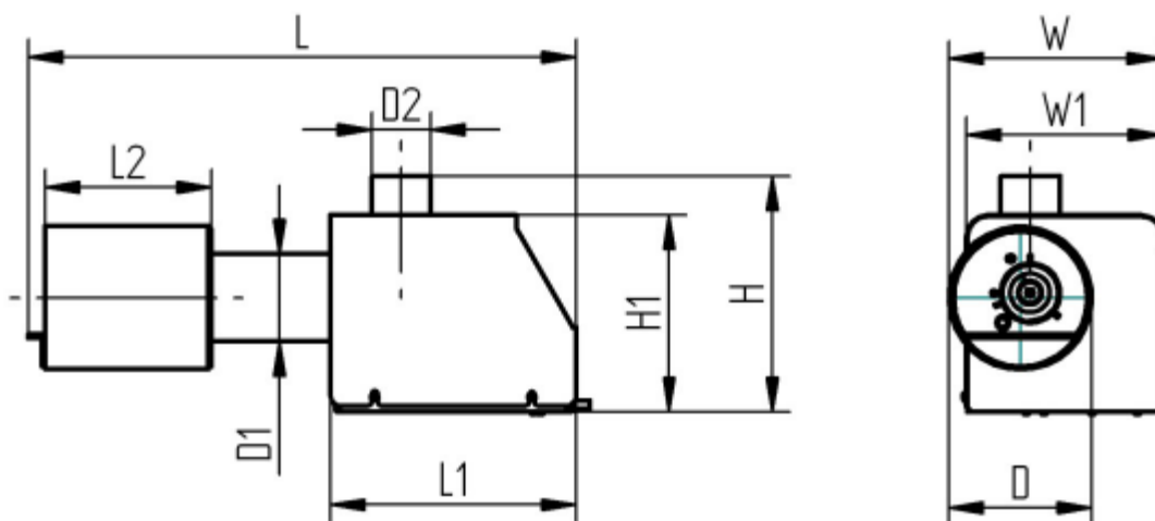
Σχήμα 2 Διαστάσεις
