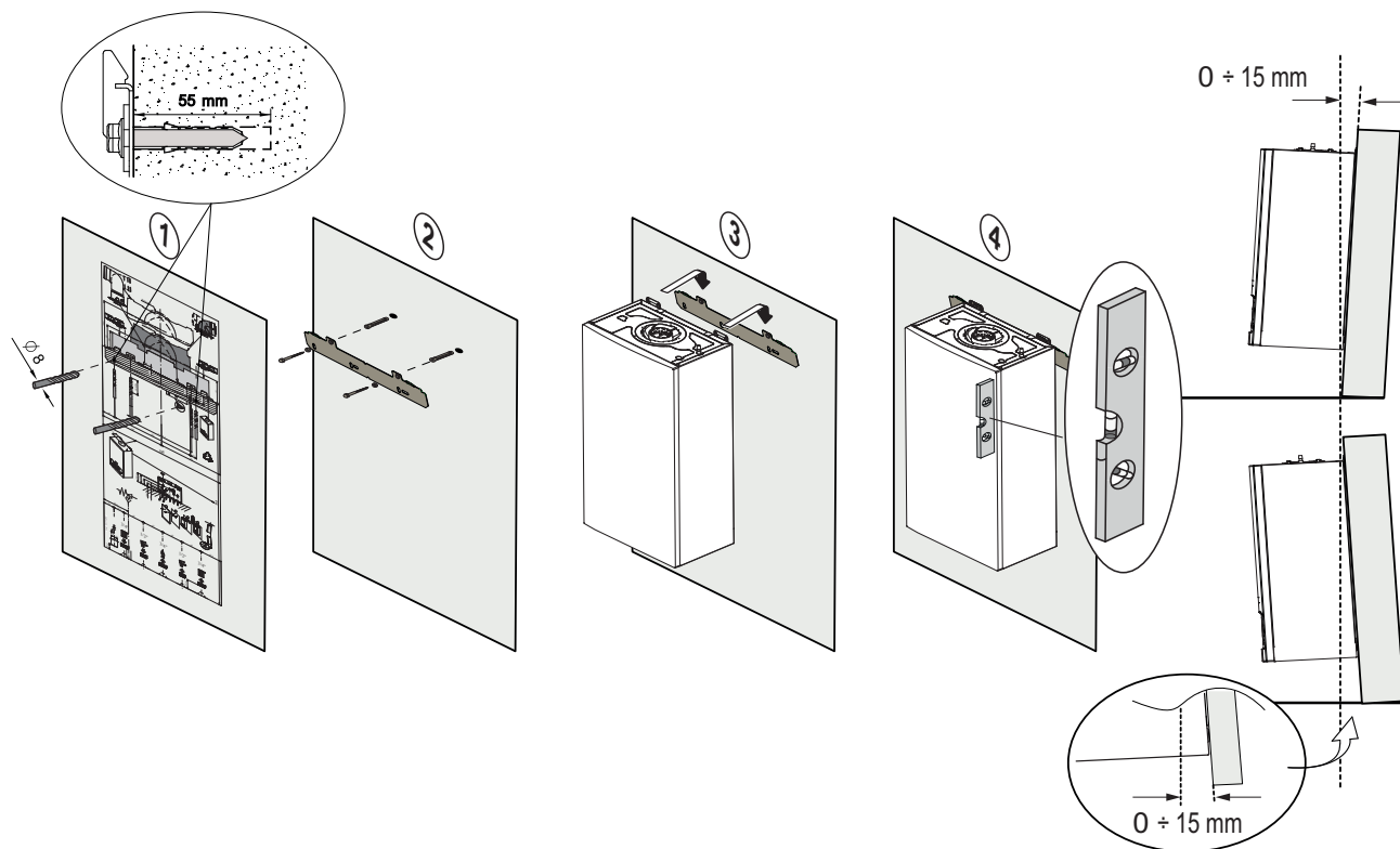
Εικ.74 Επιτοίχια εγκατάσταση
