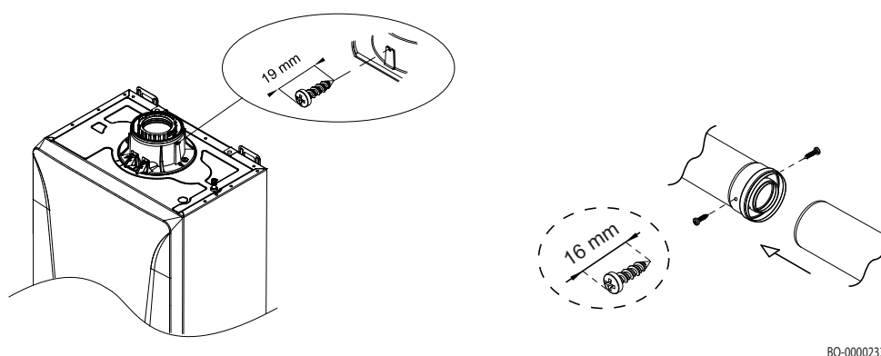
Εικ.81 Ομοαξονική στερέωση πύργου καπναερίων
