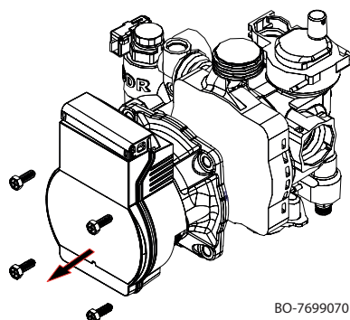
Εικ.115 Αφαίρεση μοτέρ κυκλοφορητή
