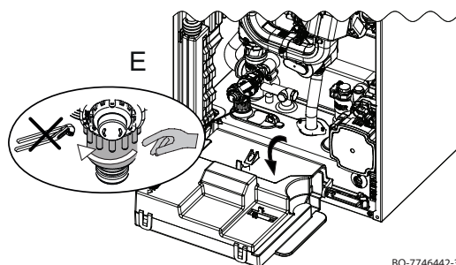
Εικ.96 Εκκένωση της εγκατάστασης
