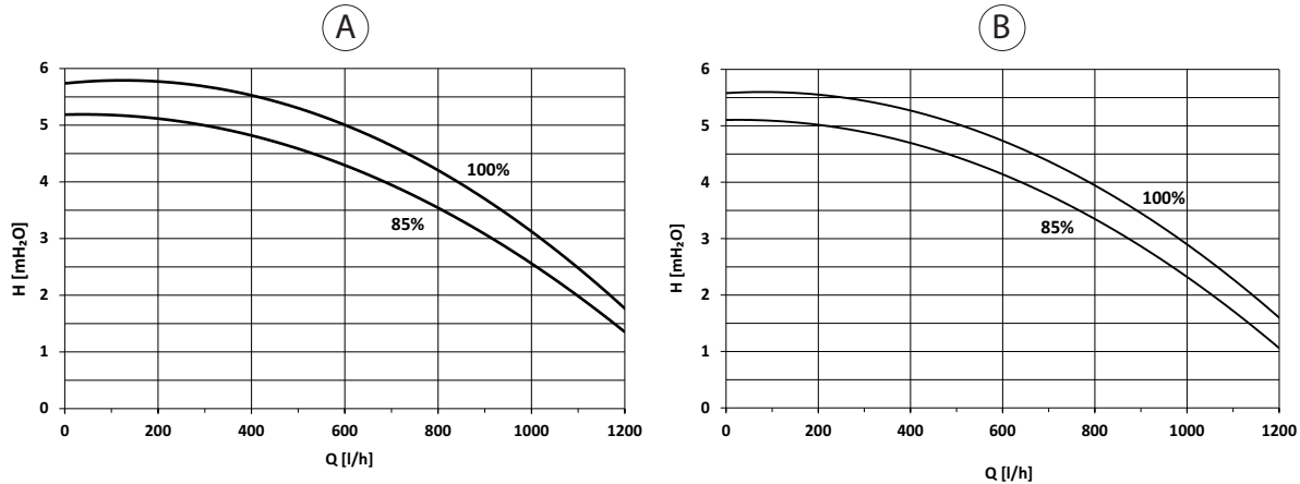
Εικ.67 Γράφημα που δείχνει το υπολειπόμενο μανομετρικό ύψος με βάση τη ροή του νερού
