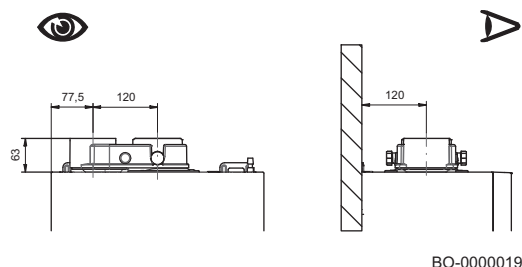
Εικ.83 Εισαγωγή-εξαγωγή διαιρούμενου τύπου
